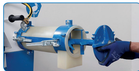
Flexibilní směšovací trubice pro jednoduché a rychlé čištění.
