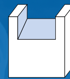
Šikmý řez pro průchod krokve
